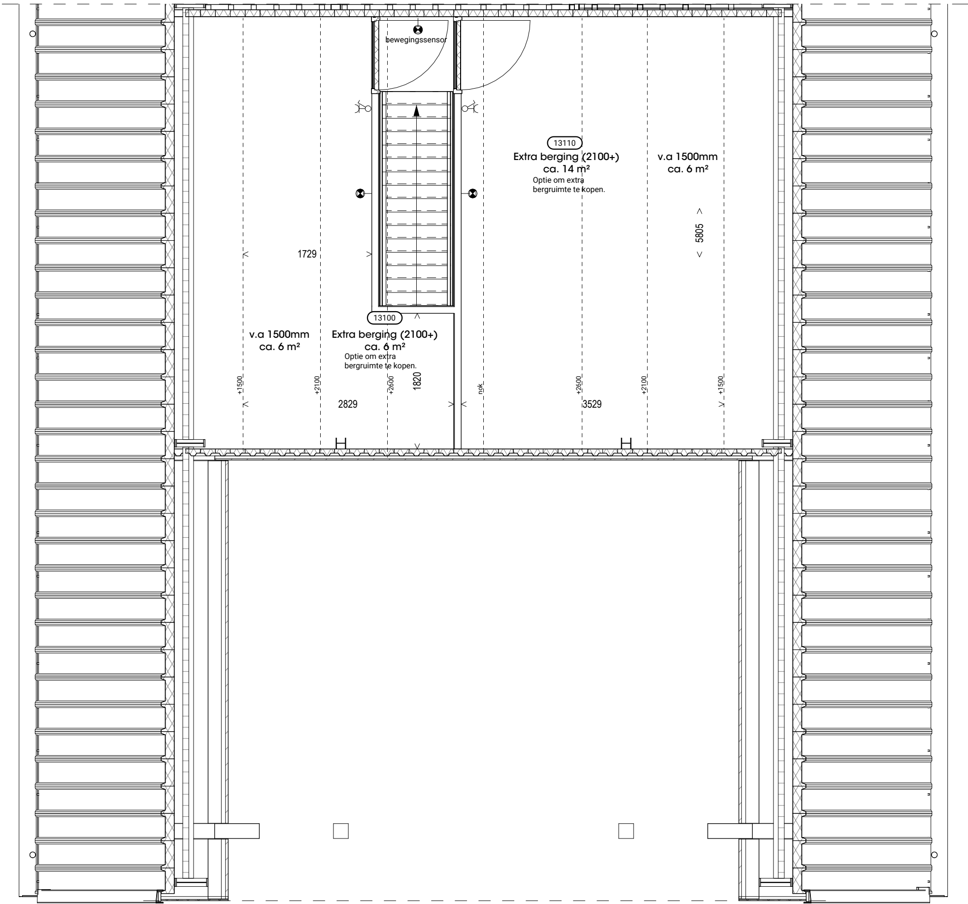
1e VERDIEPING
