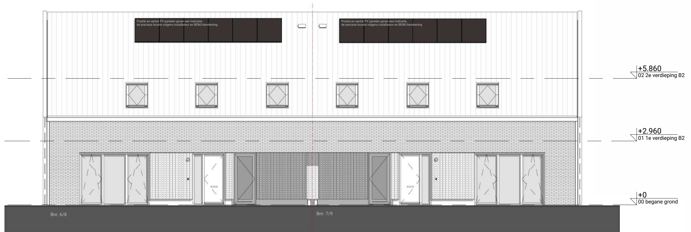
VOORGEVEL
