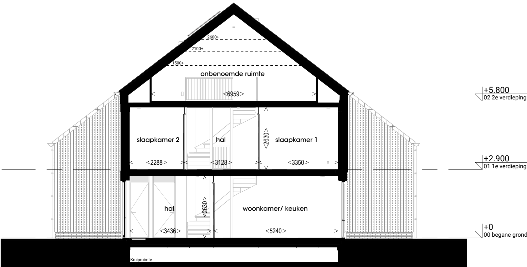
Blok 1 - Doorsnede 2
