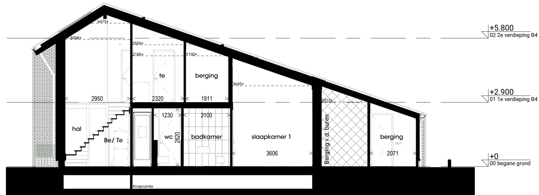
Blok 4 - Doorsnede 1
