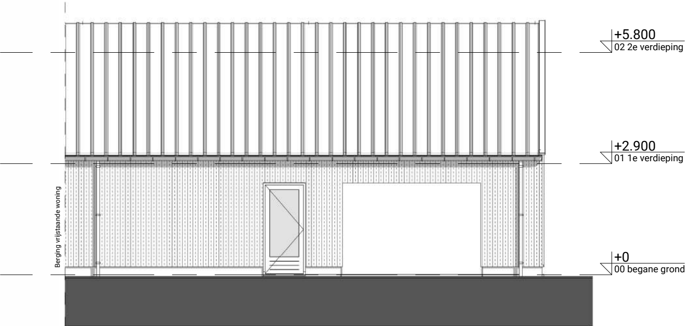
LINKER ZIJGEVEL
