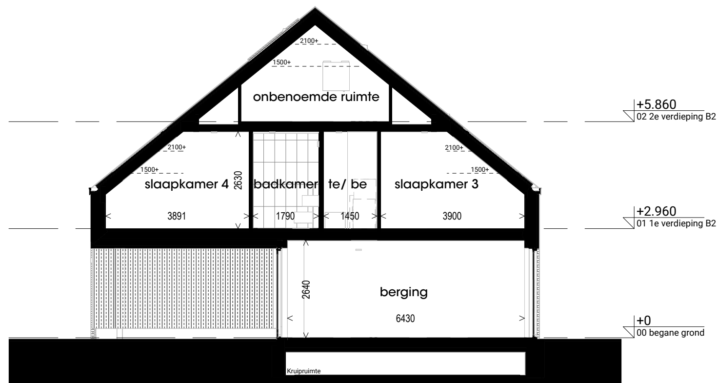
Blok 2 - Doorsnede 2
