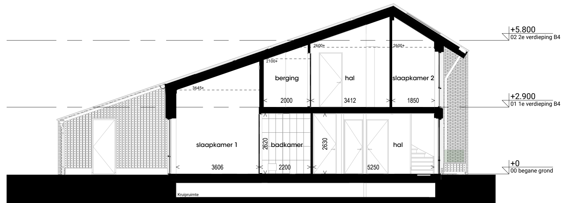
Blok 4 - Doorsnede 2
