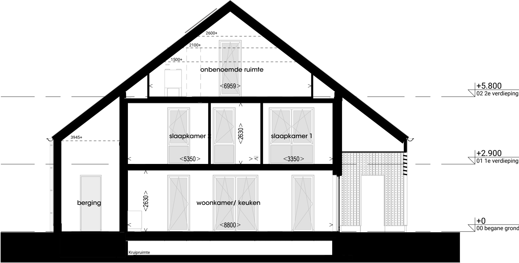
Blok 1 - Doorsnede 1
