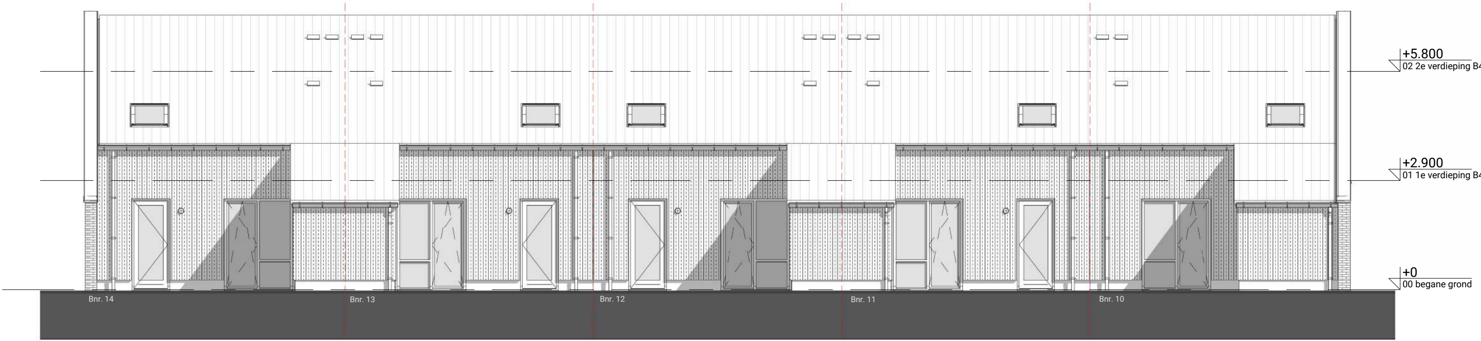
ACHTERGEVEL
