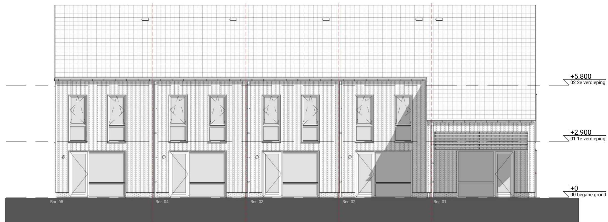
ACHTERGEVEL
