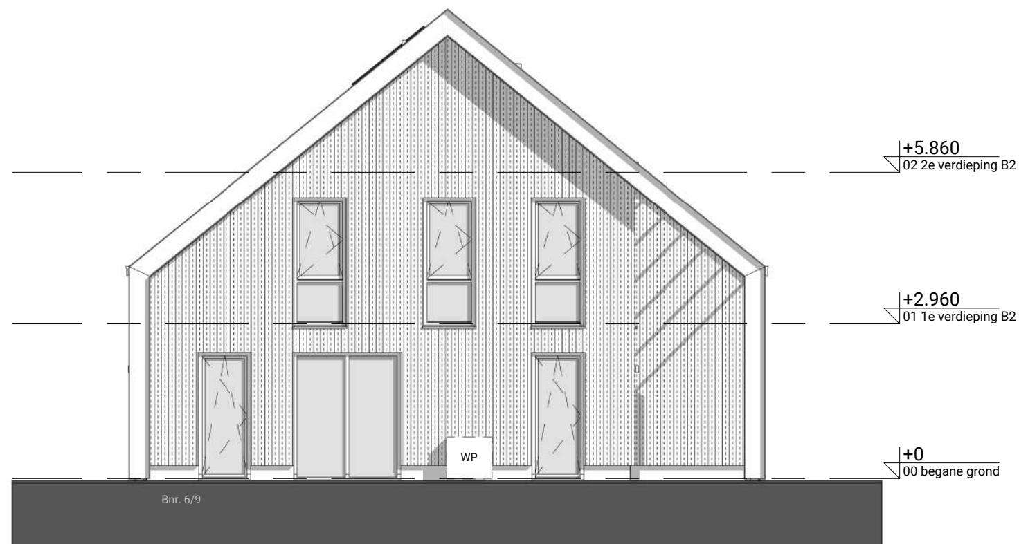
ZIJGEVEL
