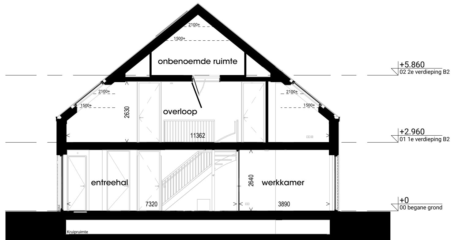
Blok 2 - Doorsnede 1
