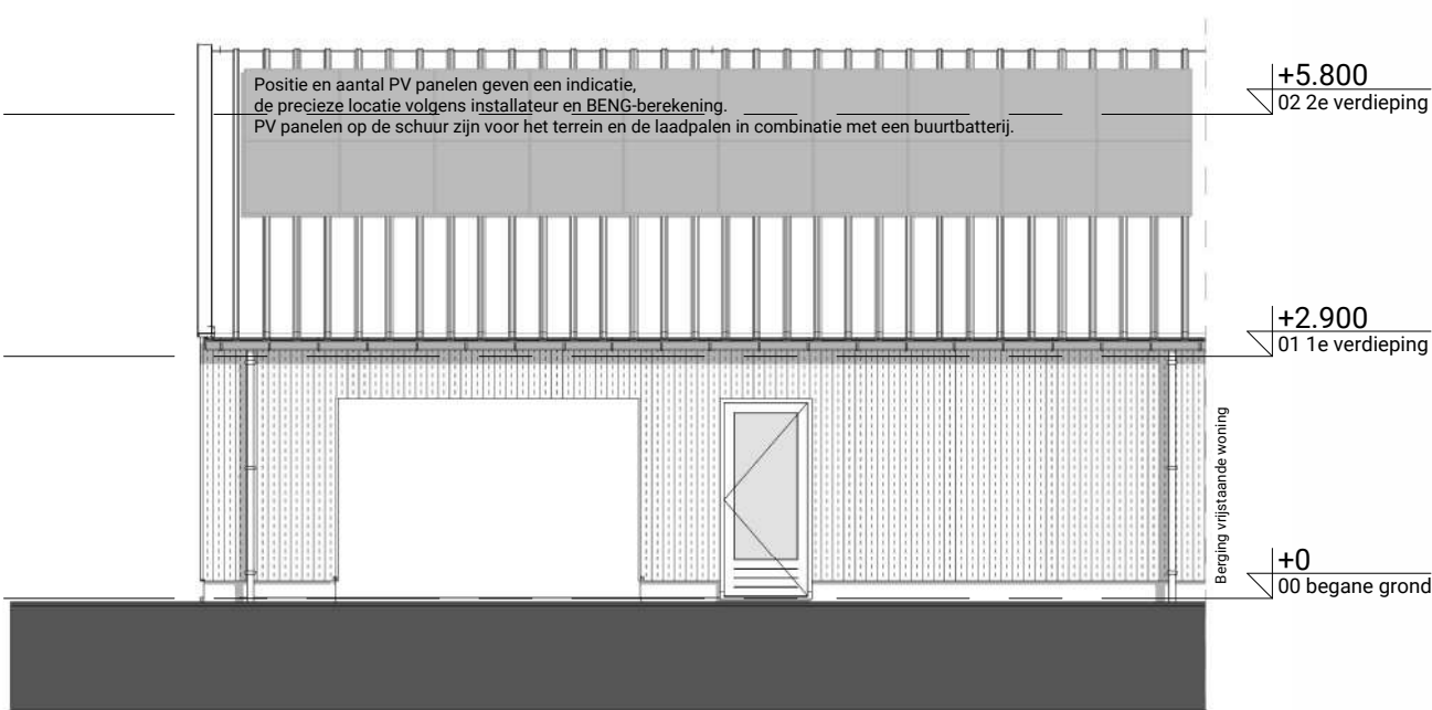
RECHTER ZIJGEVEL
