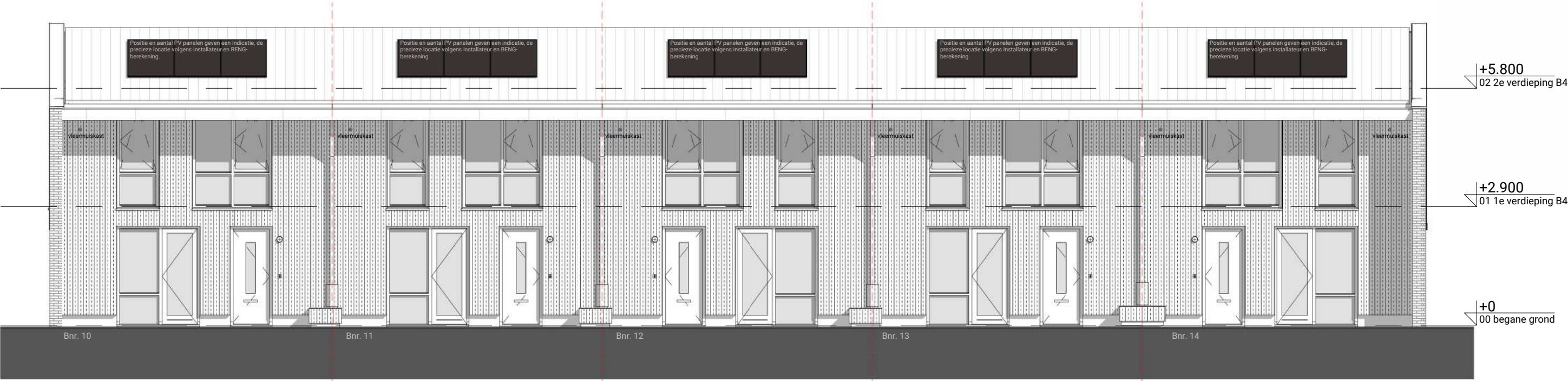
VORGEVEL
